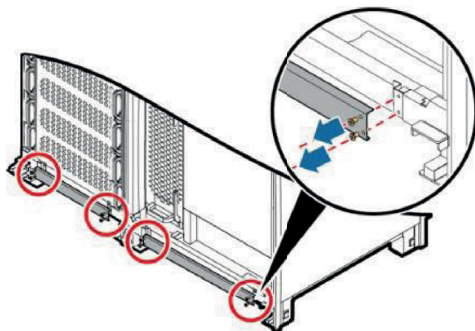
Рис. 2-56 Снятие передней перегородки (500 кВ)
